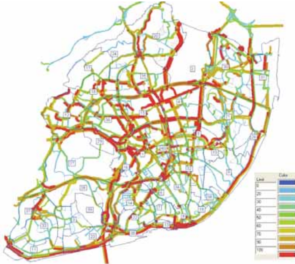
91. Níveis de saturação (%/sentido) na rede viária actual-HPT
