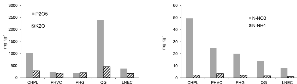
Figura 4.11 – Macronutrientes no solo
