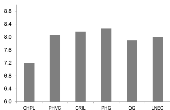
Figura 4.6 – pH do solo
