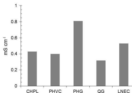
Figura 4.7 – Condutividade elétrica dos solos
