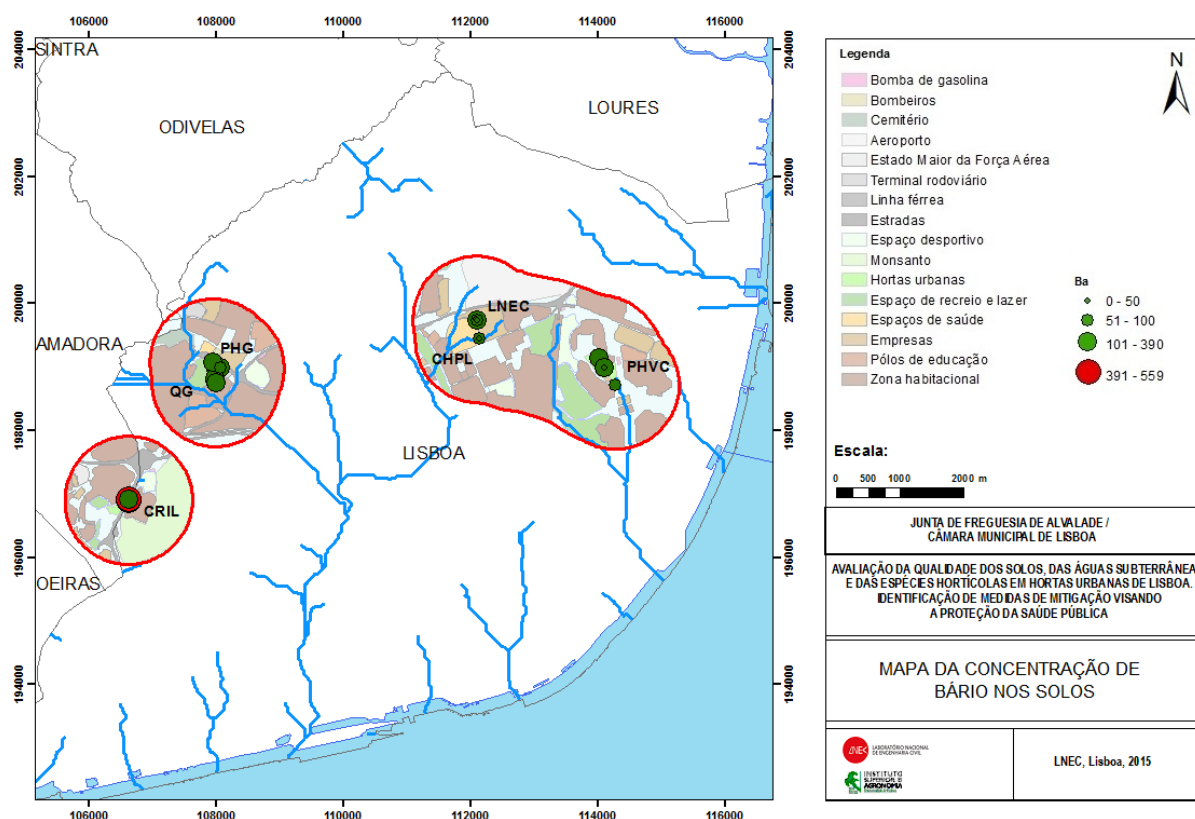
Figura 5.4 – Mapa da concentração de bário nos solos (mg/kg)
