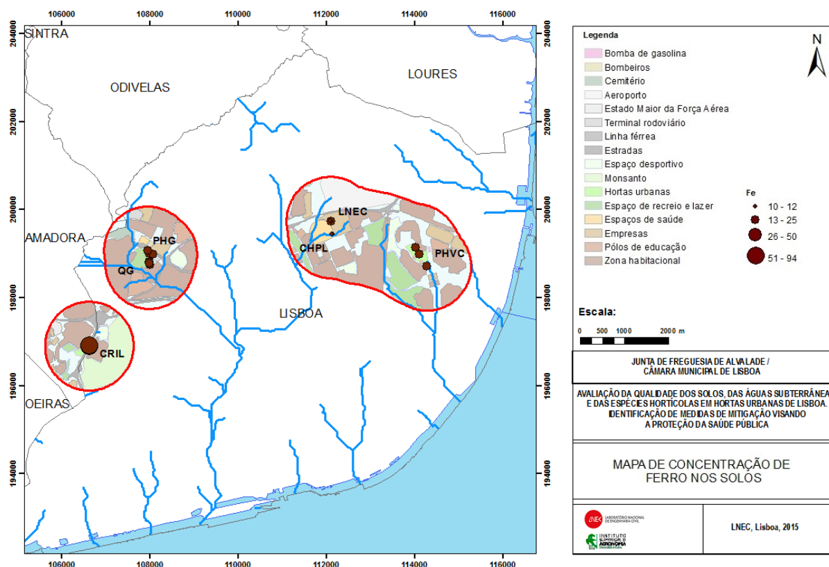
Figura 5.12 – Mapa da concentração de ferro nos solos (g/kg)
