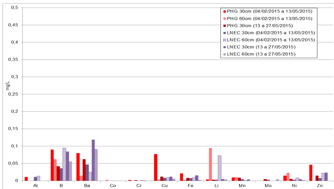
Figura 6.1 – Concentração em metais nas águas da zona vadosa do solo
