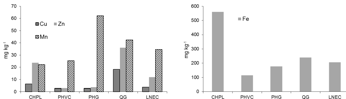
Figura 4.12 – Concentração de micronutrientes no solo
