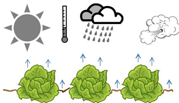
Fig. A.12. Factores climáticos que afetam a evapotranspiração das culturas
