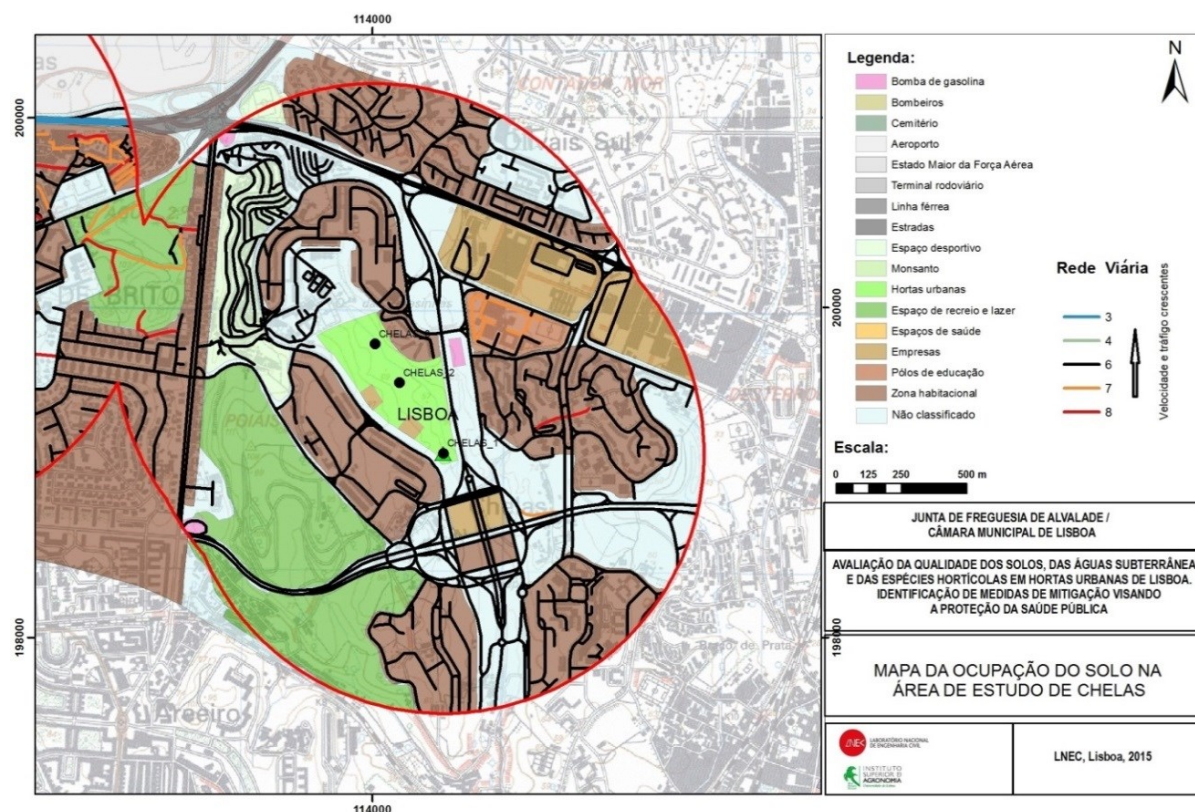
Figura 4.17 – Mapa da ocupação do solo na área de estudo do PHVC
