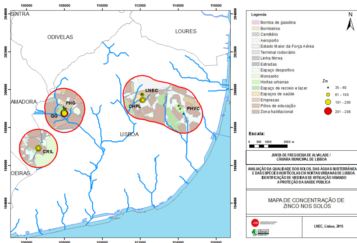
Figura 5.10 – Mapa da concentração de zinco nos solos (mg/kg)
