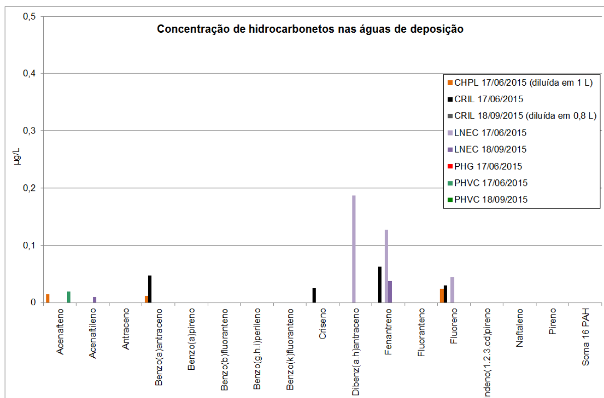
Figura 4.20 – Concentração em hidrocarbonetos nas águas de deposição atmosférica
