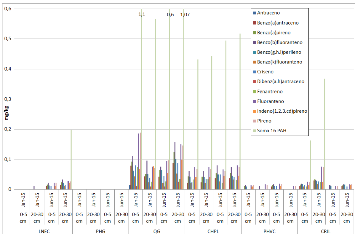
Figura 5.14 – Mapa da concentração de hidrocarbonetos nos solos (mg/kg), por local de amostragem
