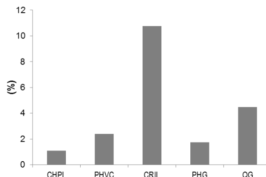
Figura 4.8 – Teor de carbonatos
