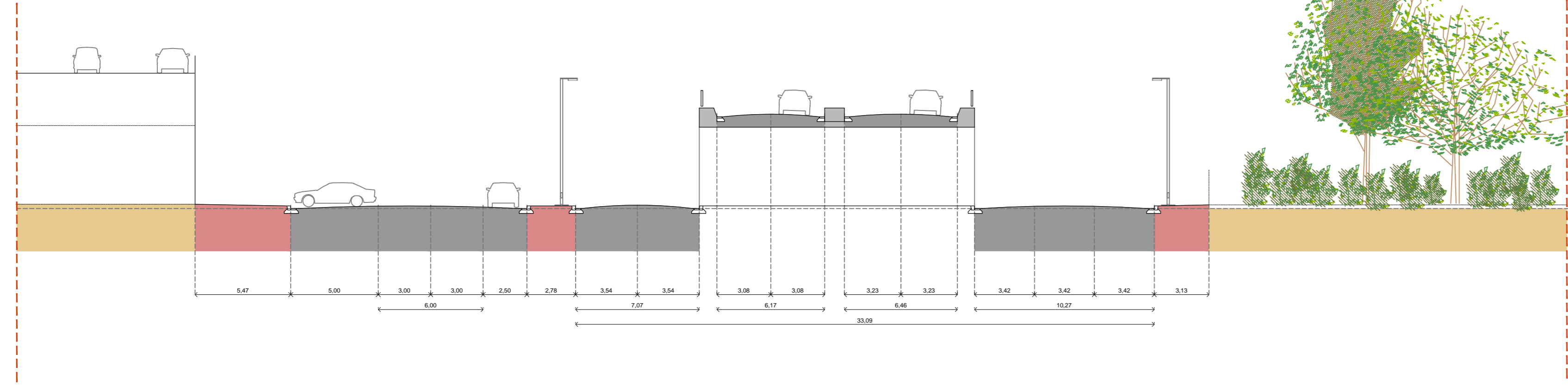
Perfil 04 - Actual
