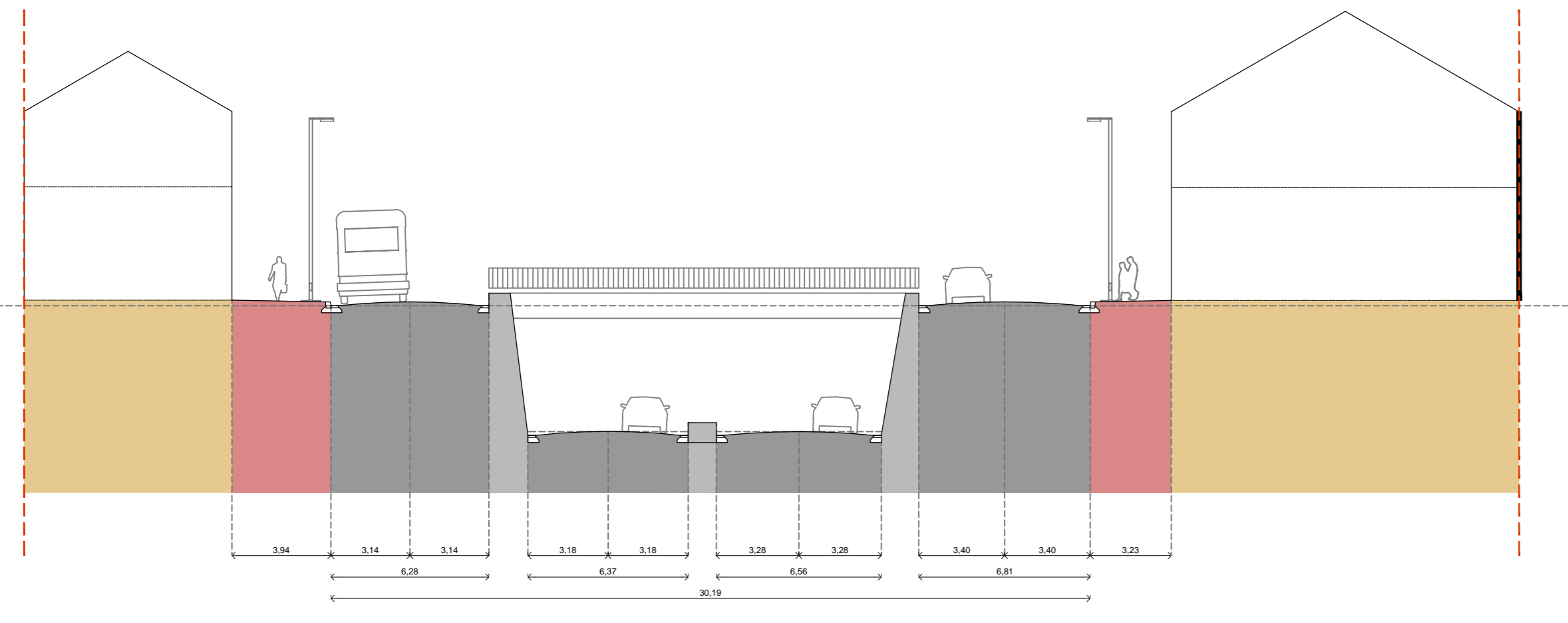
Perfil 03 - Actual
