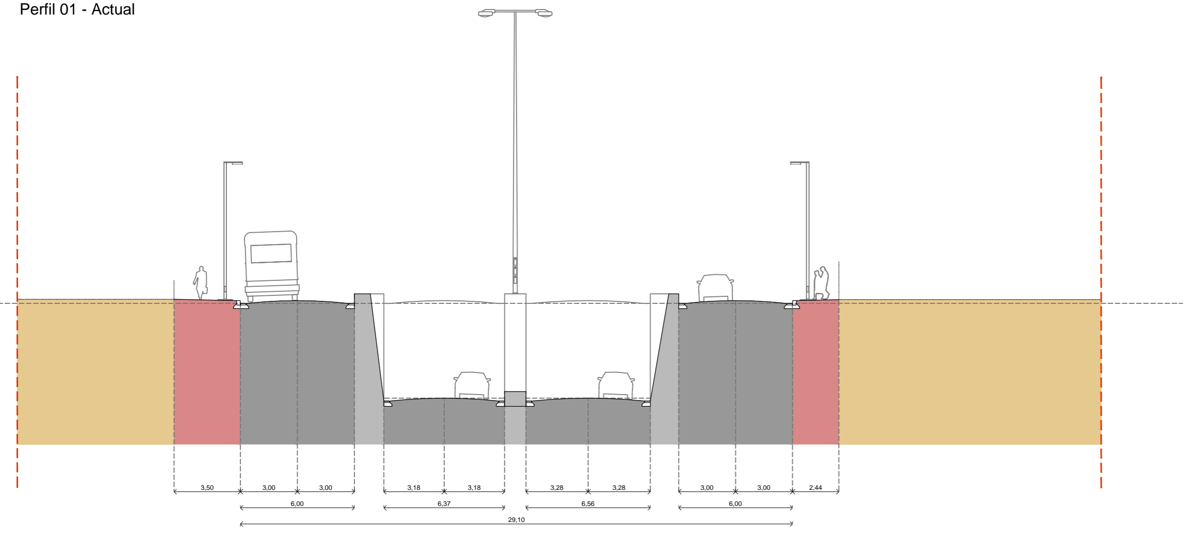
Perfil 01 - Actual
