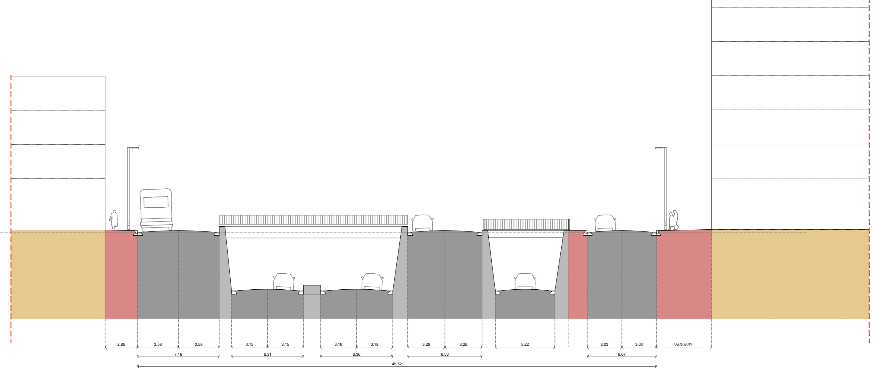
Perfil 05 - Actual
