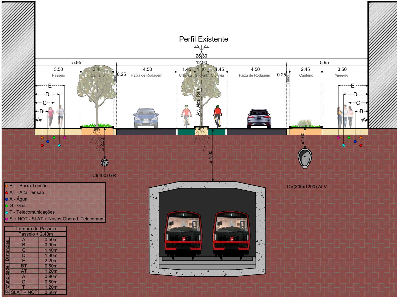
Perfil 5 (R da Palma Km 0 + 897m)
