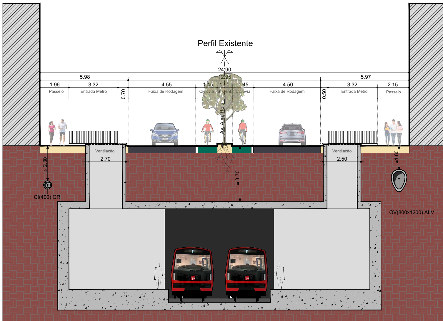
Perfil 3 (R da Palma Km 0 + 757m)
