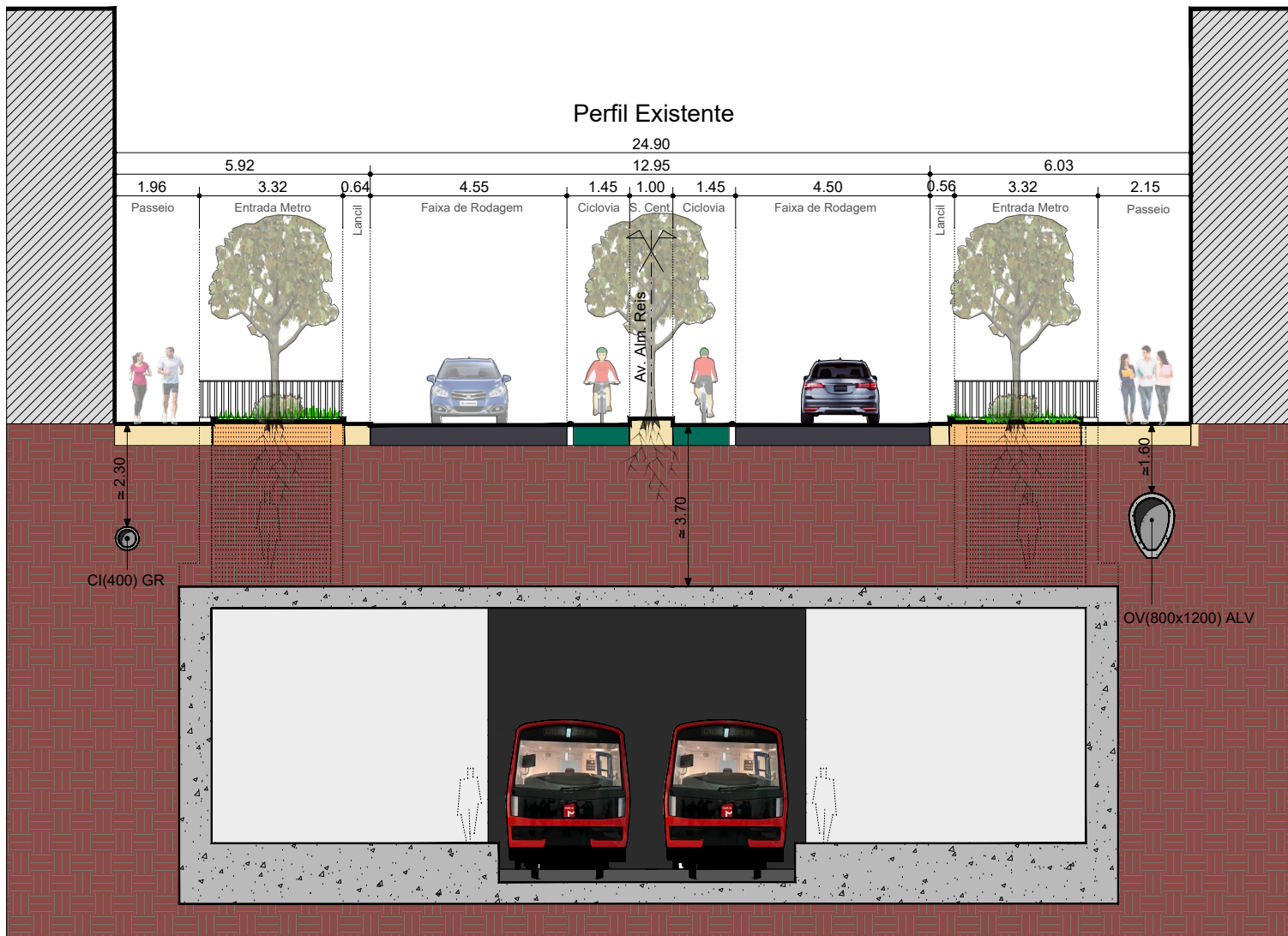
Perfil 4 (R da Palma Km 0 + 762m)
