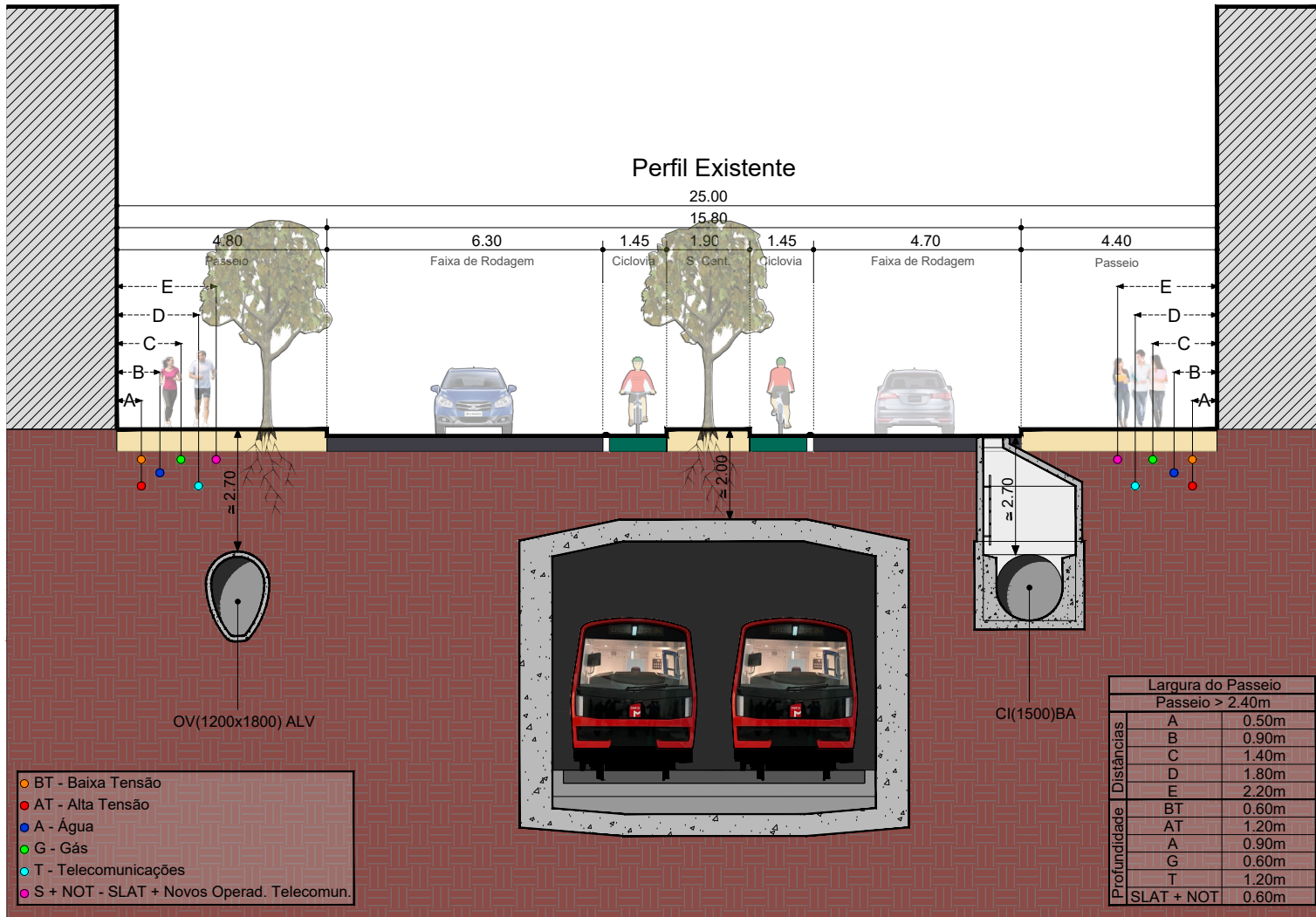
Perfil 6 (R da Palma Km 0 + 2063m)
