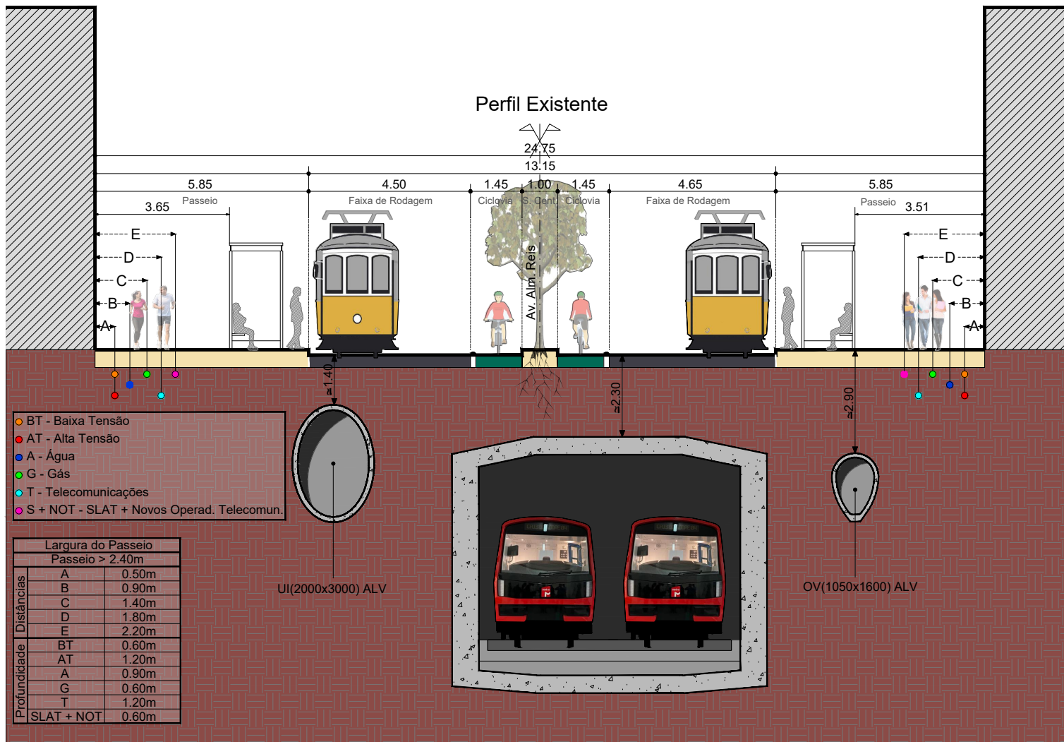
Perfil 1 (R da Palma Km 0 + 234m)
