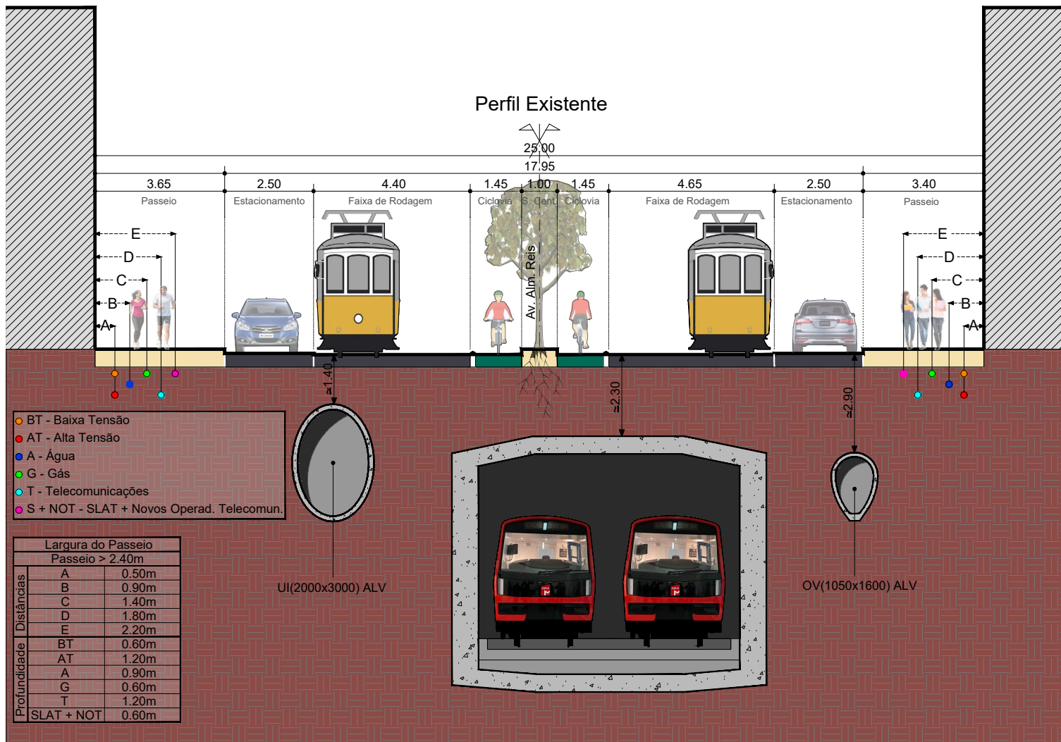
Perfil 2 (R da Palma Km 0 + 509m)
